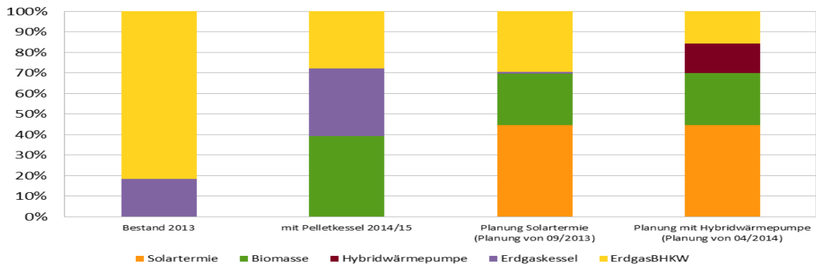
Verteilung der Wärmebereitstellung nach Primärenergie
