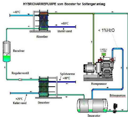
Funktionsdiagramm einer Hybrid-Wärmepumpe Quelle: Projektvorschlag vom 4.5.2014 (Planenergi), S.10
